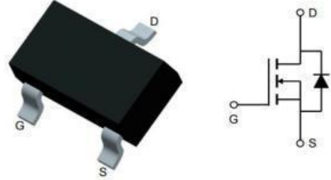
SOT23-3L
